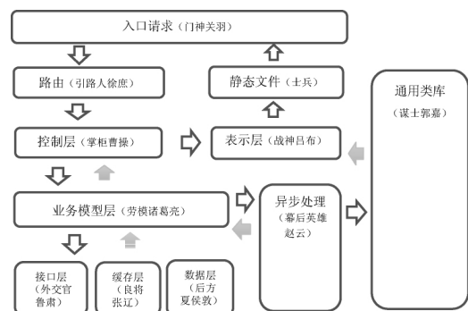
图 1 一个 Web 应用架构中的隐喻
