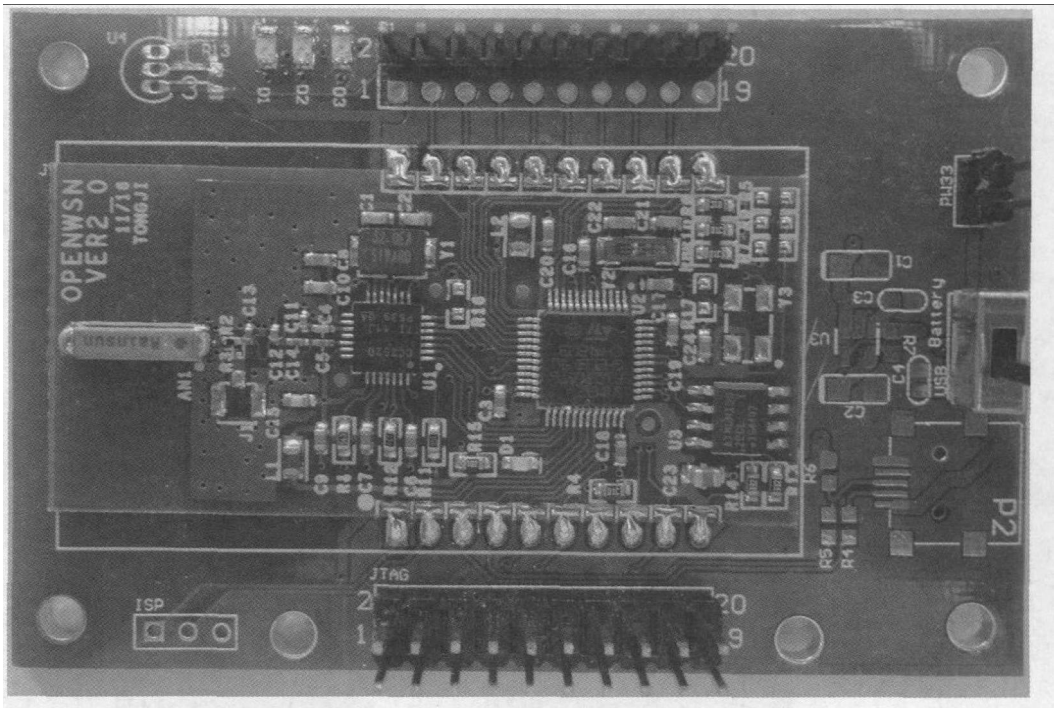
图 1: 无线传感器结点实物图
