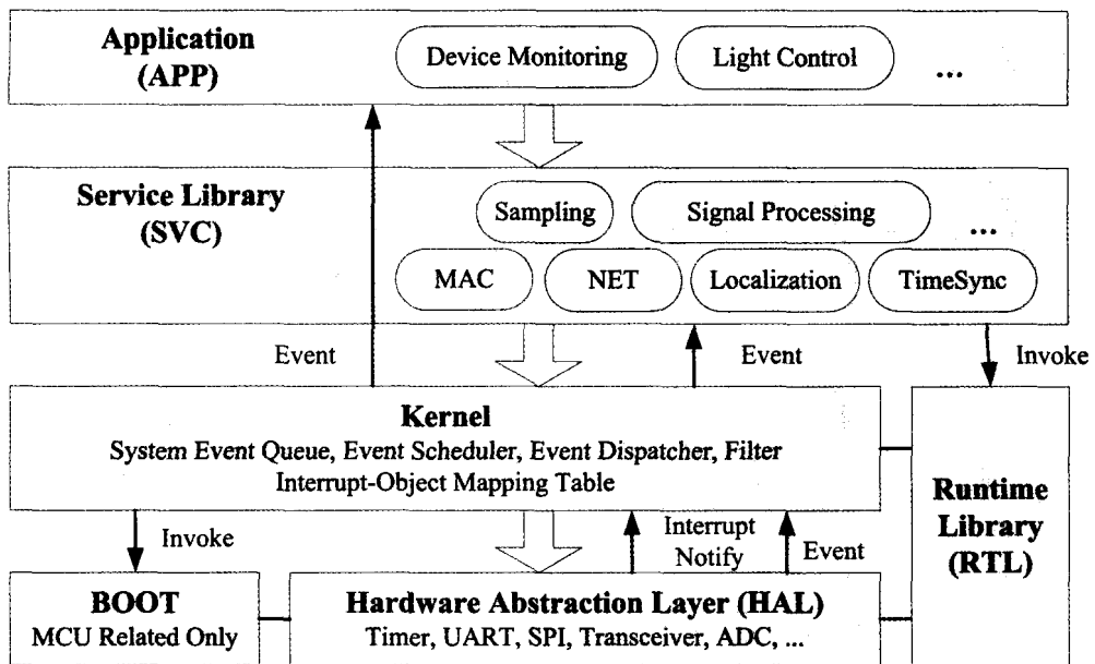
图 2: OpenWSN 平台的内部架构
